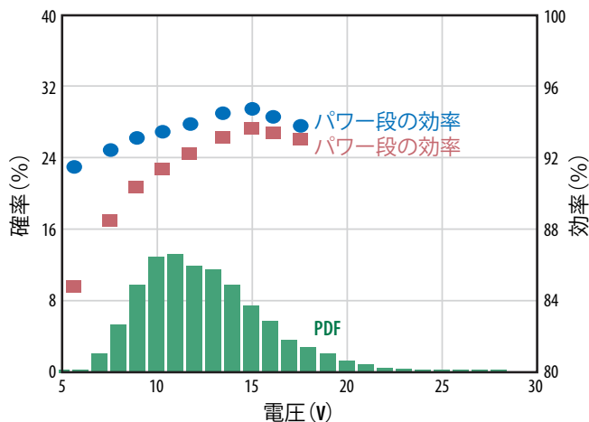
デモ・ボード定常状態のパワー一段の効率と全体の効率を測定: 20 MHzのLTE包絡線信号の確率分布 (PDF)
