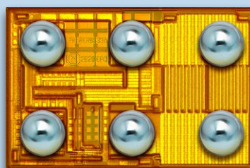
eToF™ レーザー・ドライバIC: EPC21601
