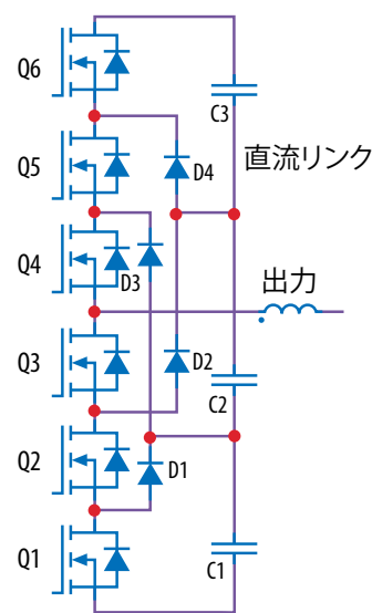
図2: 4レベルのハーフブリッジ構成
