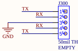
optional UART connector
